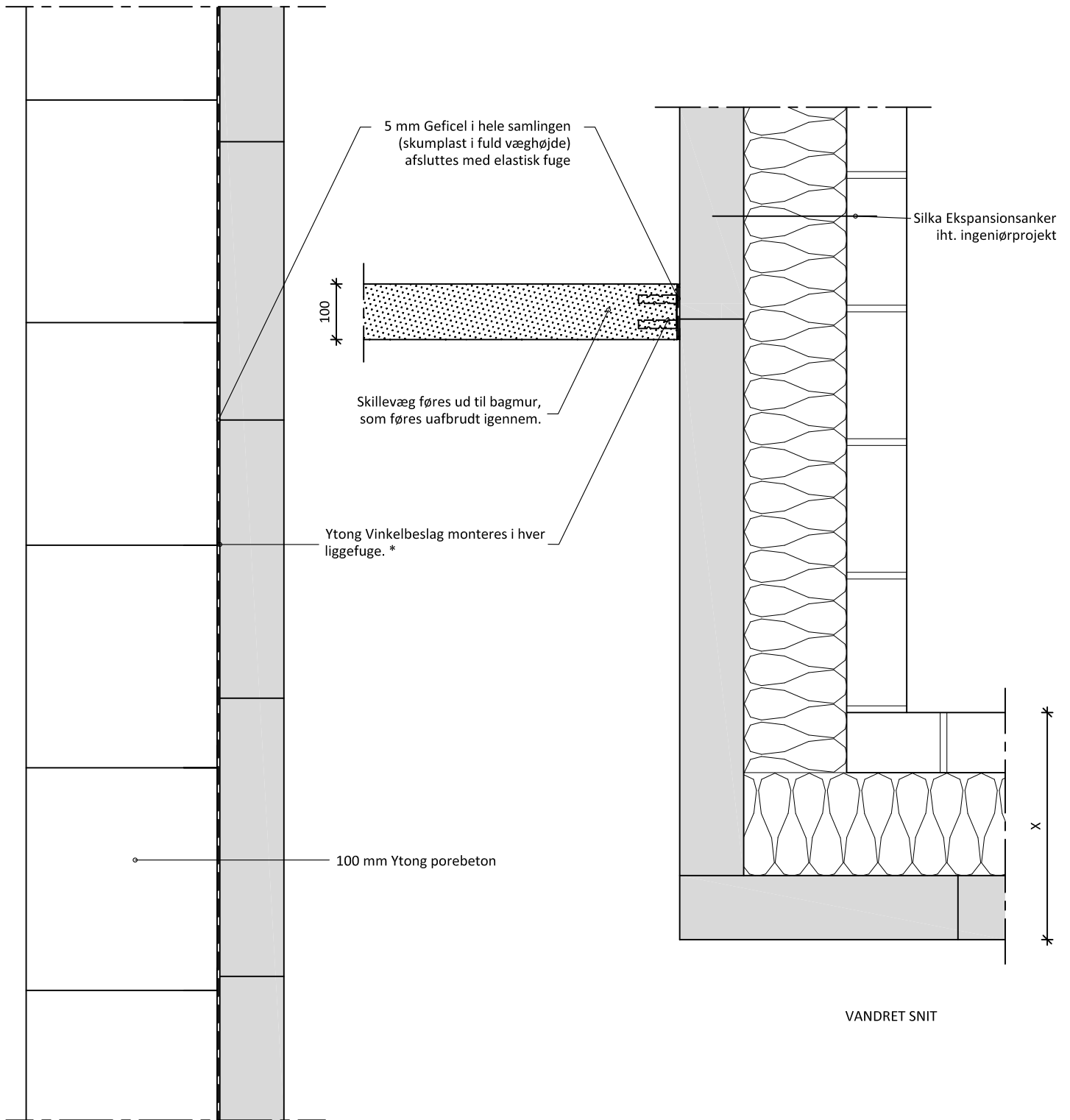
LODRET SNIT
